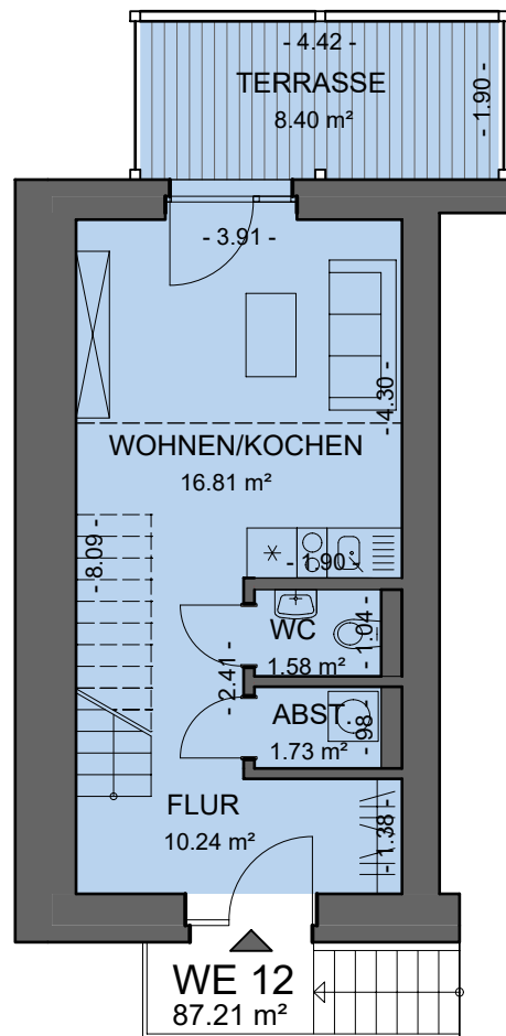
1.OBERGESCHOSS
